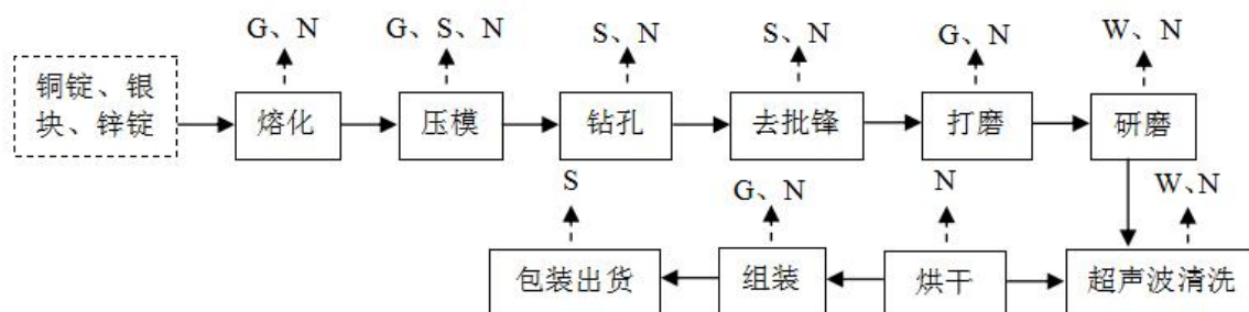
图 3-2 五金饰品生产工艺及产污环节图
