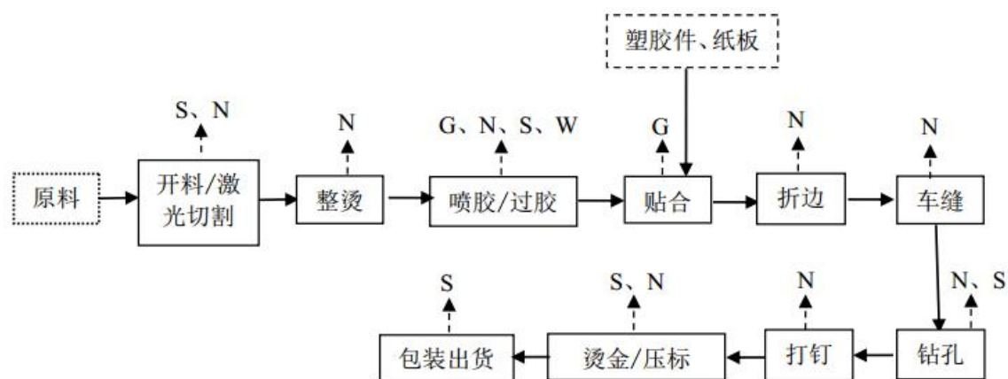
图 3-3 项目皮盒、木盒、皮具礼品生产工艺及产污环节流程图
